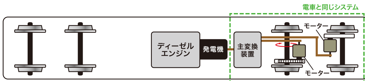
電気式気動車システムのイメージ
